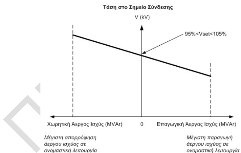
Σχεδιαγράμμα 3: Χαρακτηριστική Τάσης – Άεργου Ισχύος για ρύθμιση της Τάσης στο Σημείο Σύνδεσης .
