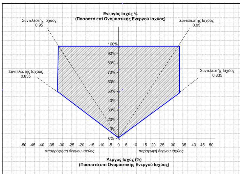
Σχεδιάγραμμα 2β: — Ελάχιστη υποχρεωτική περιοχή λειτουργίας του Αιολικού Πάρκου για Ενεργό Ισχύ και Άεργο Ισχύ (ελάχιστο εύρος δυνατότητας λειτουργίας). Η Ενεργός Ισχύς και η Άεργος Ισχύς μετρούνται στο Σημείο Σύνδεσης .
