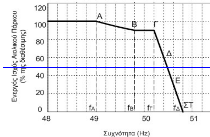
Σχεδιάγραμμα 6: Καμπύλη Συχνότητας - παραγόμενης Ενεργού Ισχύος . (Η μορφή της καμπύλης και οι τιμές των παραμέτρων για την Ενεργό Ισχύ και τη Συχνότητα θα καθορίζονται από τον ΔΣΜΚ σύμφωνα με το -Τ16.4.6.4.2.4).
