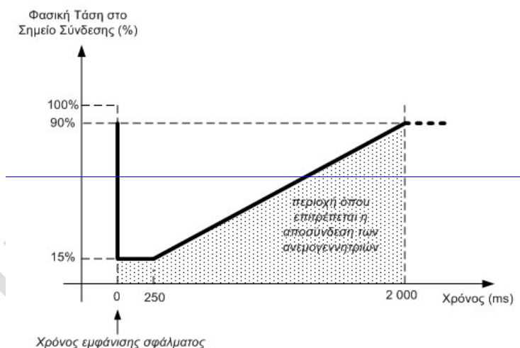
Σχεδιάγραμμα 4: Καμπύλη/Καμπύλη Τάσης για Αδιάλειπτη Λειτουργία ανεμογεννητριών.
