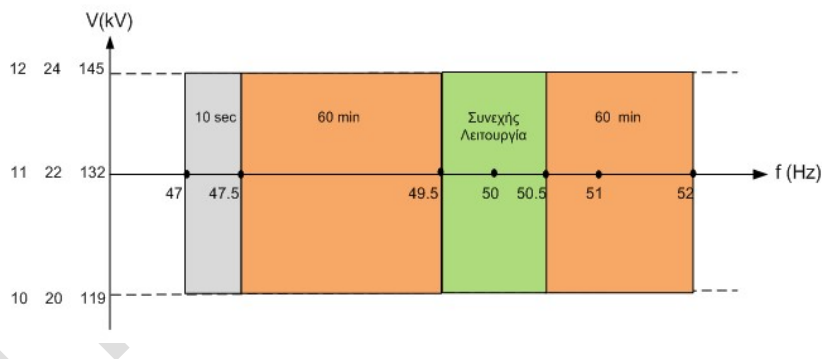
Σχεδιάγραμμα 1:- Υποχρεωτική Δυνατότητα Λειτουργίας Αιολικών Πάρκων (εντός του εύρους Τάσης κανονικής λειτουργίας του Ηλεκτρικού Συστήματος ) σε συνάρτηση με τη Συχνότητα .
