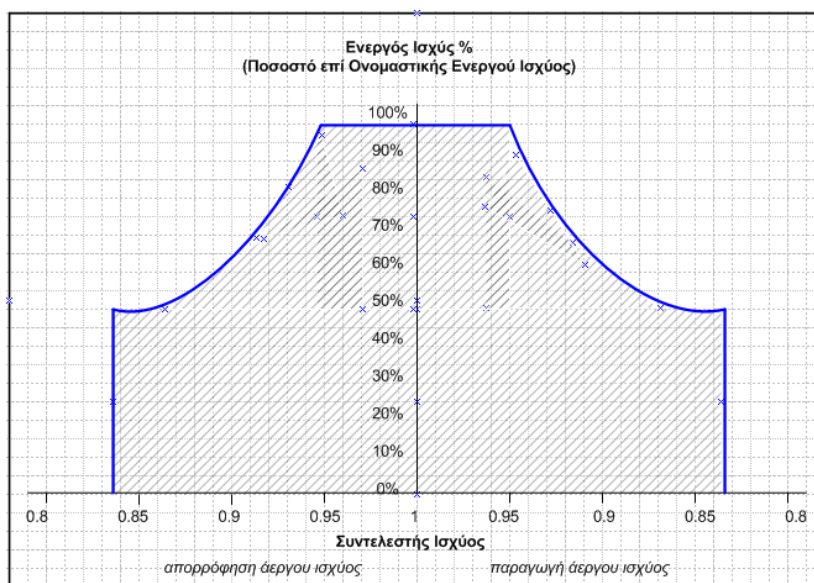
Σχεδιαγράμμα 2γ: Ελάχιστη υποχρεωτική περιοχή λειτουργίας του Αιολικού Πάρκου για Ενεργό Ισχύ και Συντελεστή Ισχύος (ελάχιστο εύρος δυνατότητας λειτουργίας). Η Ενεργός Ισχύς και ο Συντελεστής Ισχύος μετρούνται στο Σημείο Σύνδεσης .
