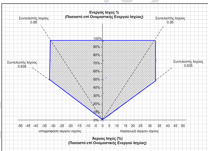
Σχεδιάγραμμα 2β: Ελάχιστη υποχρεωτική περιοχή λειτουργίας του Αιολικού Πάρκου για Ενεργό Ισχύ και Άεργο Ισχύ (ελάχιστο εύρος δυνατότητας λειτουργίας). Η Ενεργό Ισχύς και η Άεργος Ισχύς μετρούνται στο Σημείο Σύνδεσης .
