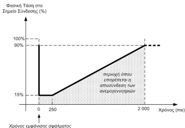
Σχεδιάγραμμα 4: Καμπύλη Τάσης για Αδιάλειπτη Λειτουργία ανεμογεννητριών.
