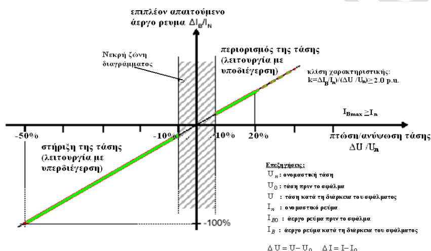
Σχεδιαγράμμα 5: Άεργο ρεύμα εξόδου κατά τη διάρκεια μεγάλων μεταβολών της Τάσης.
