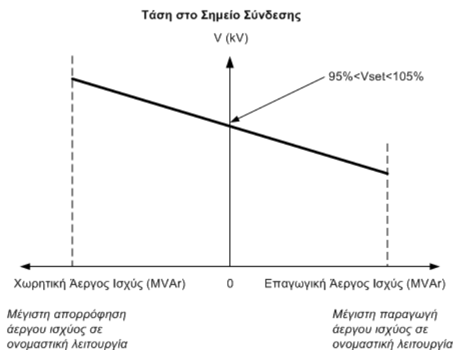
Σχεδιαγράμμα 3: Χαρακτηριστική Τάσης – Άεργου Ισχύος για ρύθμιση της Τάσης στο Σημείο Σύνδεσης .
