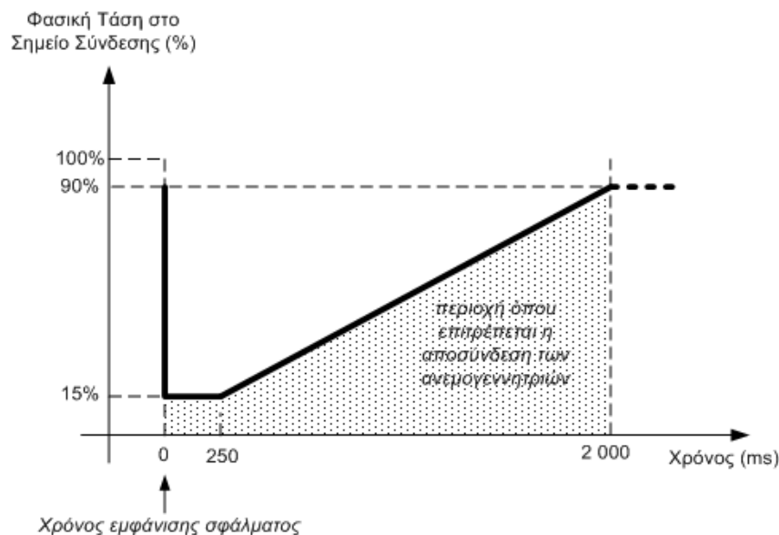
Σχεδιαγράμμα 4: Καμπύλη Τάσης για Αδιάλειπτη Λειτουργία ανεμογεννητριών.
